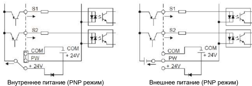
Рис 4.18 PNP режим
