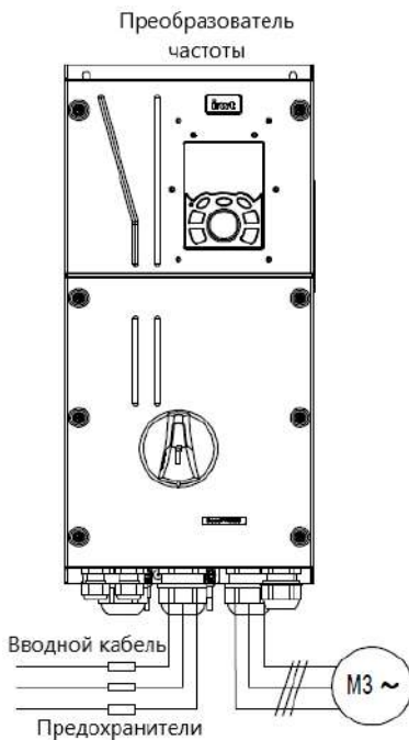
Рис 4.19 Подключение предохранителей
