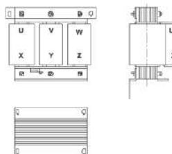
Выходной реактор
