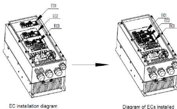
Рис А-1 ПЧ 7,5 кВт или выше с установленными платами расширения
