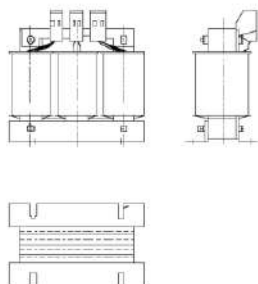
Входной реактор
