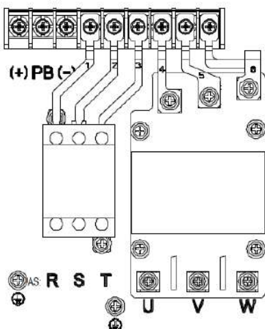
Рис 4.8 Силовые клеммы 004G/5R5P–5R5G/7R5P
