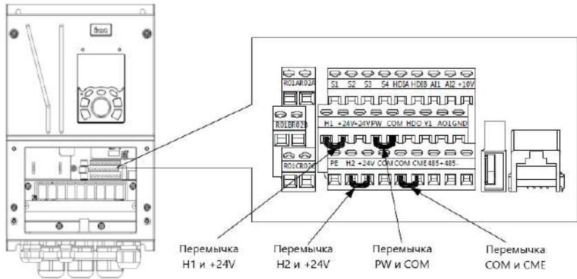
Рис 4.16 Расположение U-образных контактов
