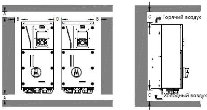
Рис 4.4 Параллельная установка
