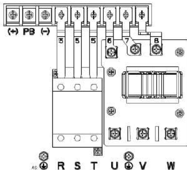
Рис 4.10 Силовые клеммы 018G/022P–022G/030P
