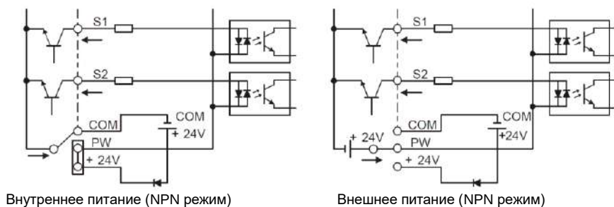
Рис 4.17 NPN режим
